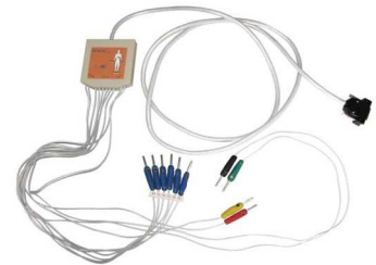
CABOS PACIENTE PARA ECG compatíveis com todos os fabricantes e modelos
